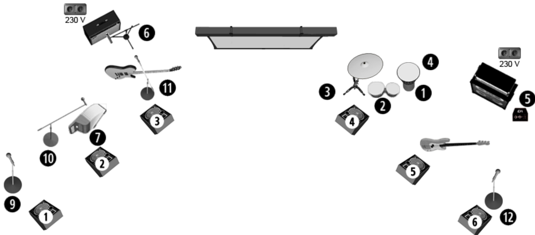
Entre Images et Mots Stage Plot 2016 v1
